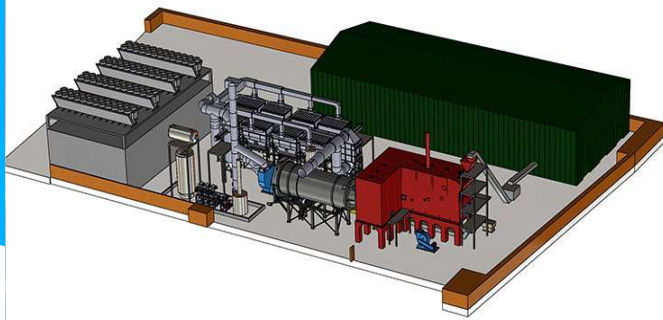
3D Module Creo V6
